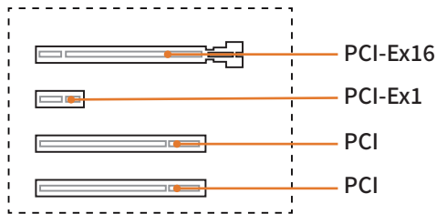
图2-4 PCI扩展插槽
