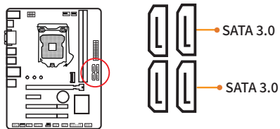
图2-10 SATA接口
