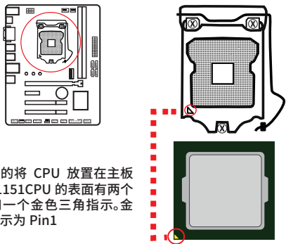
图2-7 CPU安装
