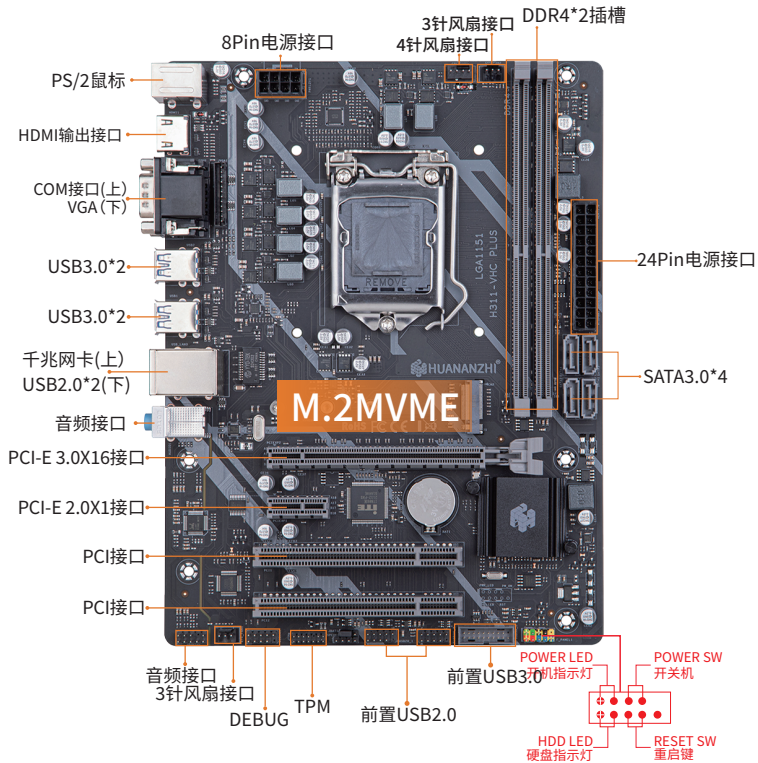
图1-1 H311-VHC PLUS主板图解
